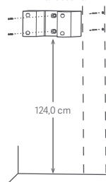
Montaż uchwyty ścienne na akcesoria
